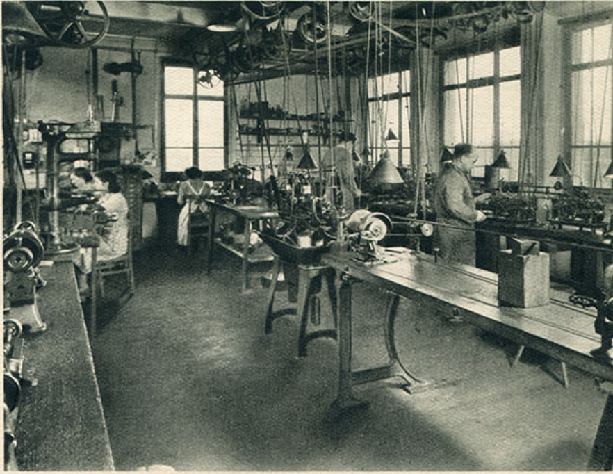
LES FONTENELLES Atelier de décolletage
