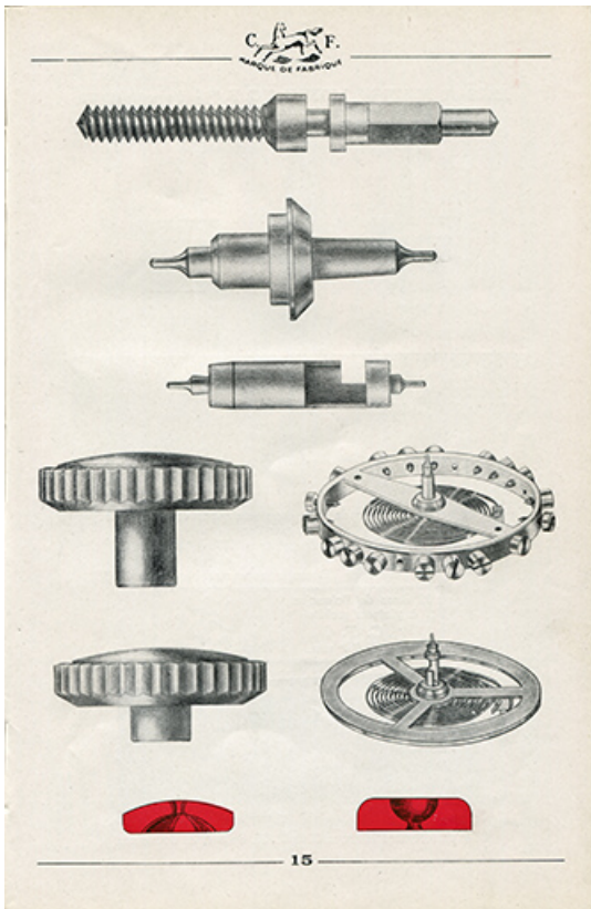
[Exemples de production de la société Cheval Frères : cylindre et axe, balancier-spiral, couronne de remontoir et rubis], 1950. 25, Maîche, 4 rue de la Gare
