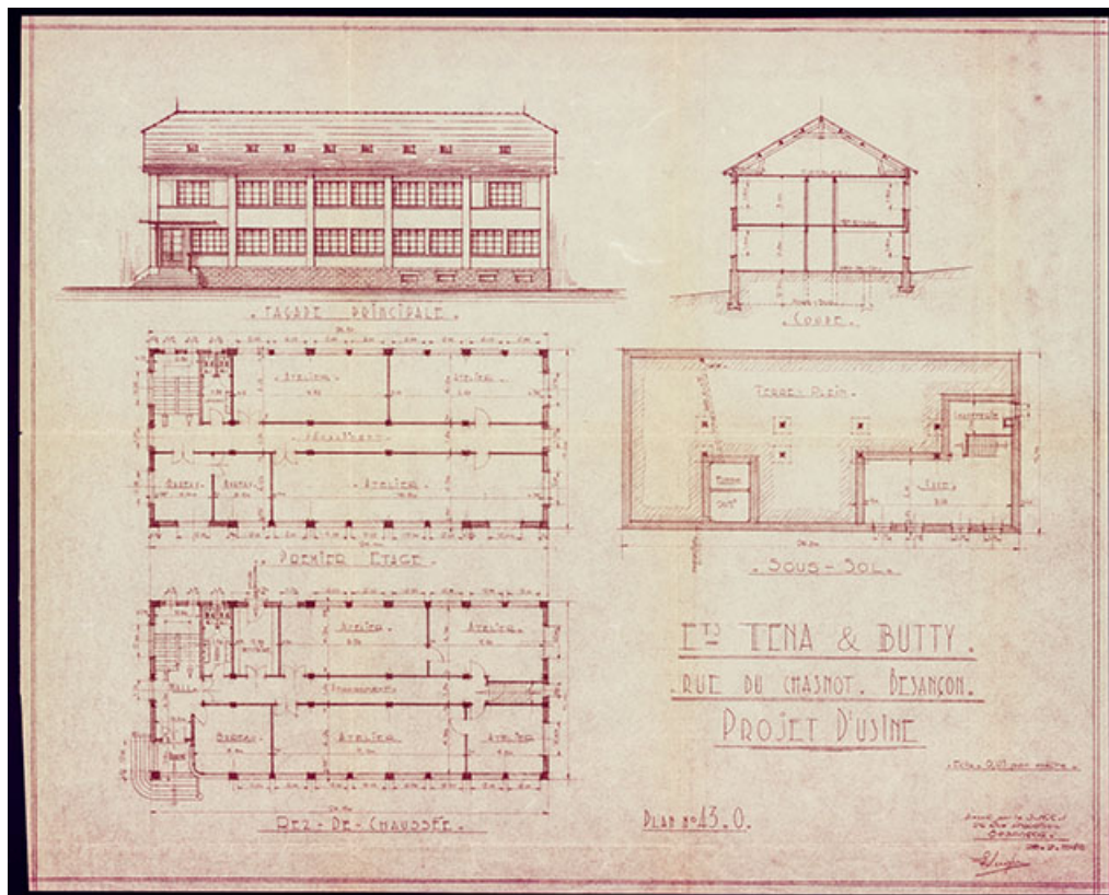
Ets Tena-Butty. Projet d'usine, 1946. 25, Besançon, 42 rue Narcisse Lanchy
