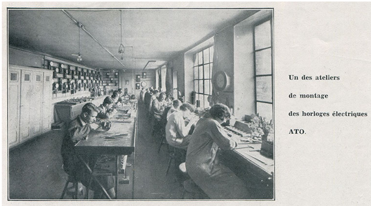
Un des ateliers de montage des horloges électriques Ato, 1933.
