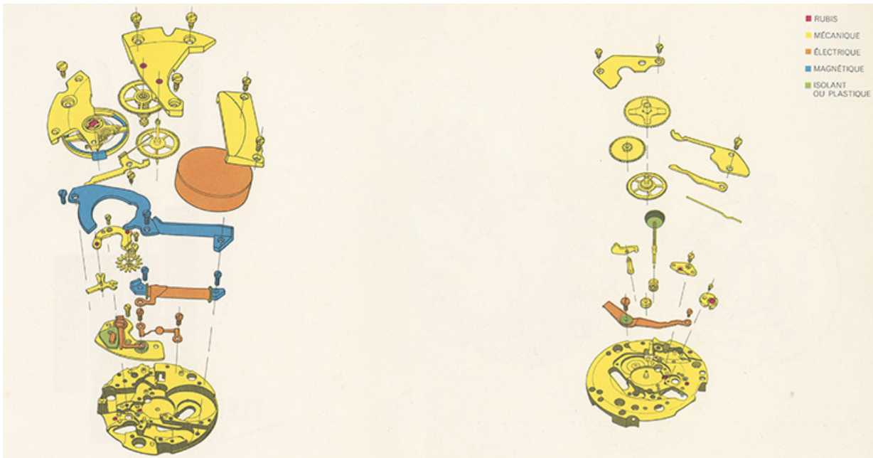
Eclaté d'un mouvement de montre Lip, 1969. 25, Besançon chemin de Palente
