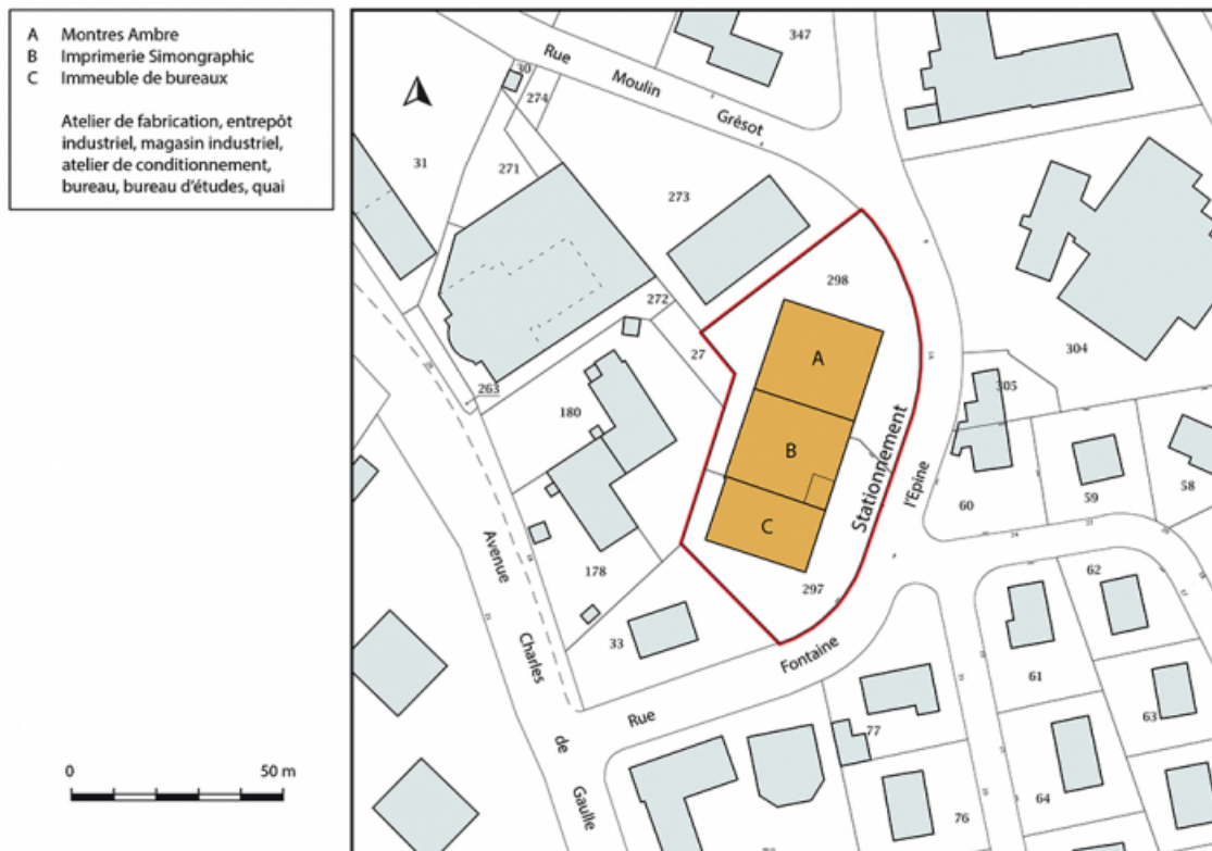
Plan-masse et de situation. Extrait du plan cadastral, 2018, section AE, 1/1 000. 25, Morteau, 1 et 1A rue Fontaine-l'Épine
