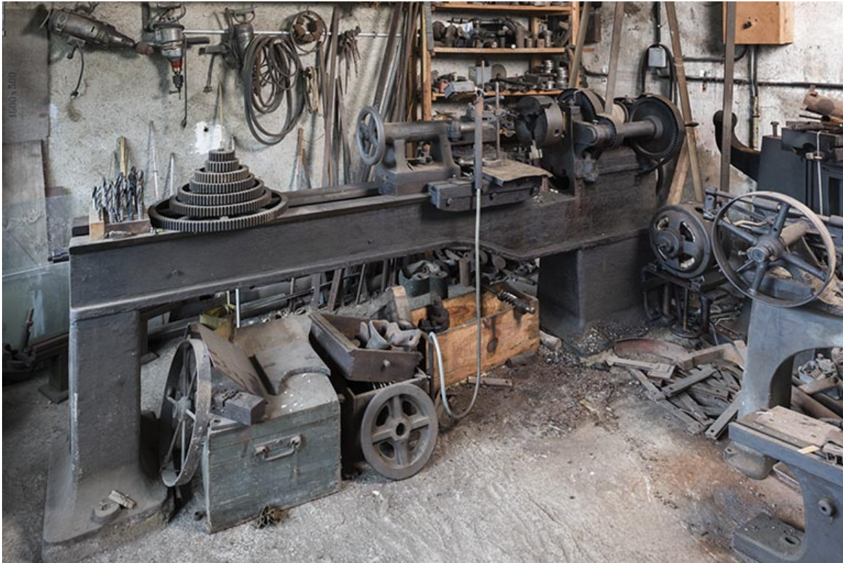
Atelier de mécanique : gros tour de mécanicien.
