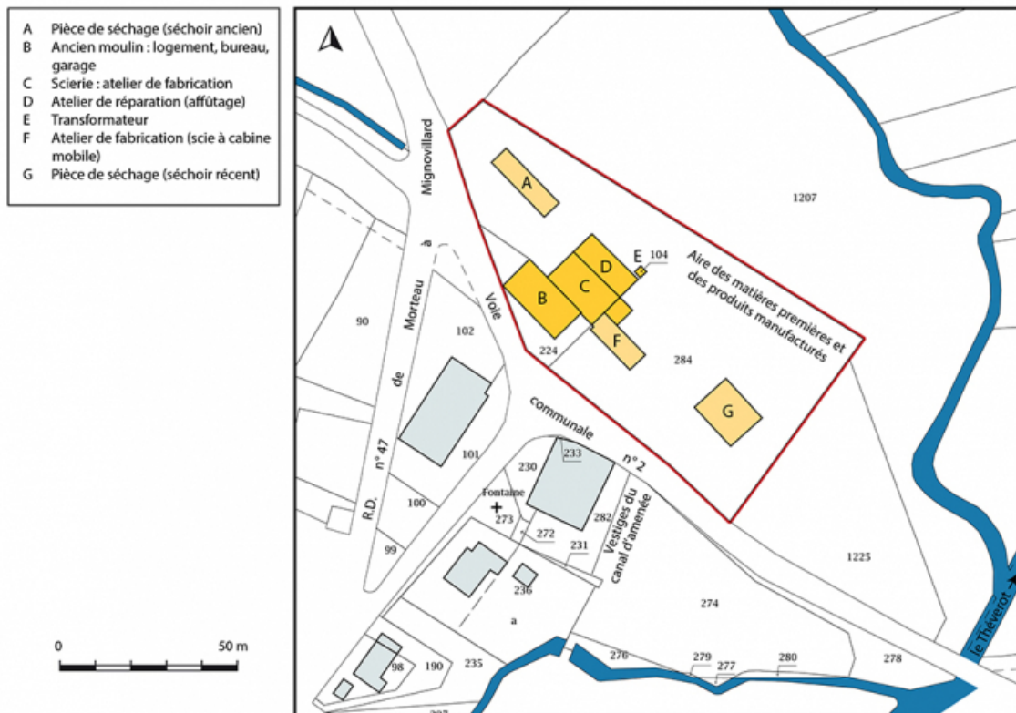
Plan-masse et de situation. Extrait du plan cadastral, 2017, section AD, 1/1 000. 25, Grand'Combe-Châteleu, lieudit : les Douffrans
