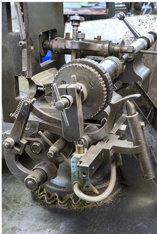
Machine à refendre les morilles : détail du système de commande (avec la fraise à refendre au second plan). 25, Grand'Combe-Châteleu, 14 rue les Grands Saules, lieudit : les Forges
