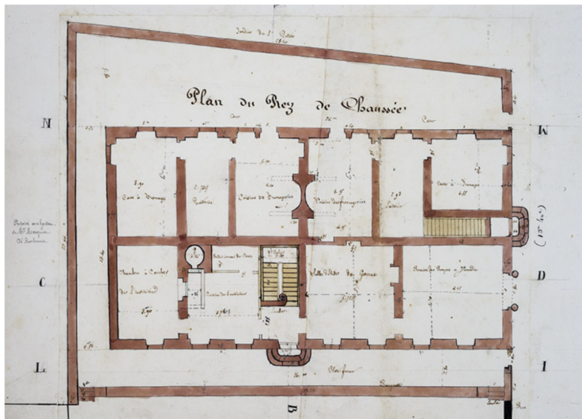
Plans, coupe et élévations du projet de construction d'une maison commune [...]. Plan du rez-de-chaussée, 1832. 25, Aubonne, 1 rue de la Mairie
