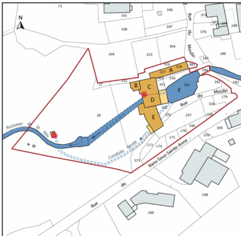
Plan-masse et de situation. Extrait du plan cadastral, 2015, section A. 25, Éternoz, 4 rue du Moulin
