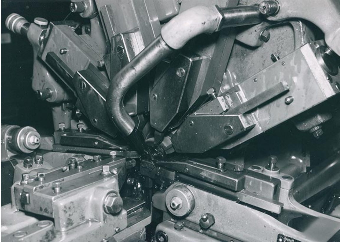
[6 burins Cardur montés sur une décolleteuse], 1978.
