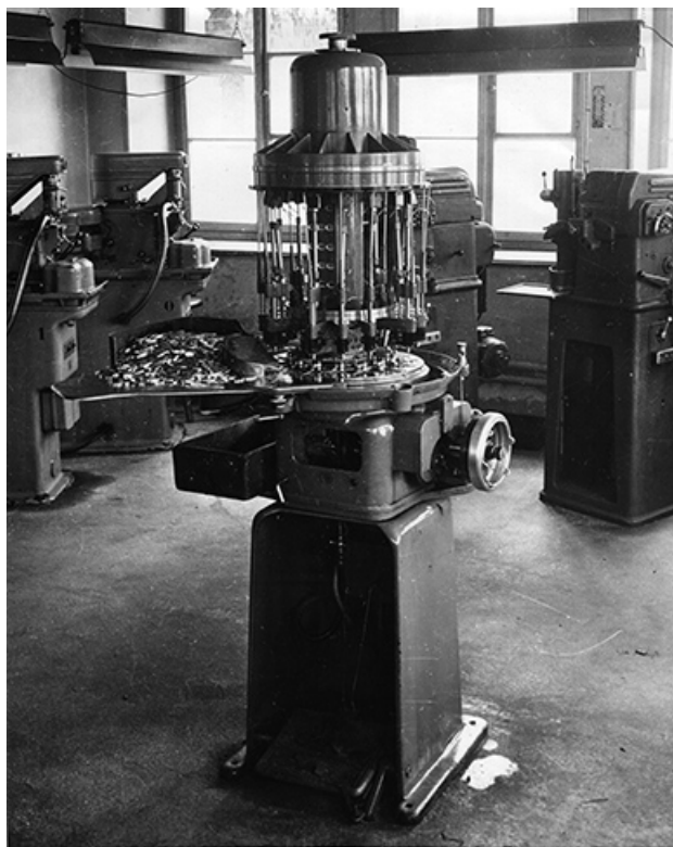
Perceuse semi-automatique multibroche auto-contrôlée à très grande production
