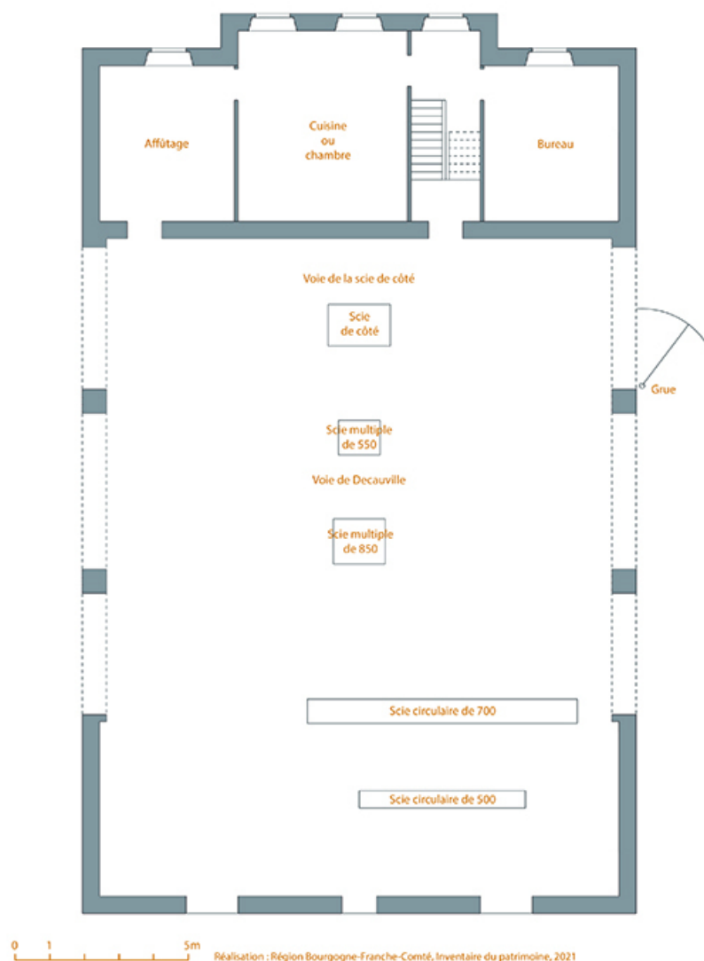
Plan du rez-de-chaussée, mise au net d'un relevé, 1/100, par E. Parrod, 1912. 25, Les Fourgs, 2 Grande-Rue
