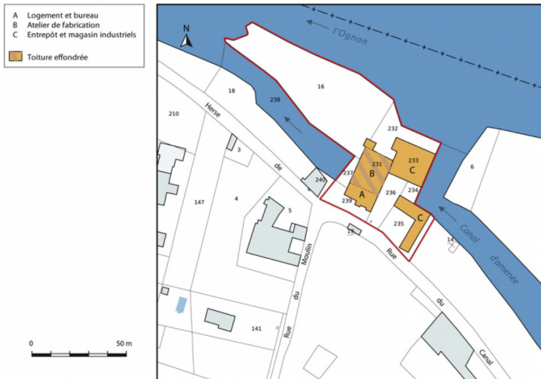
Plan-masse et de situation. Extrait du plan cadastral, 2015, section AB. 25, Cussey-sur-l'Ognon, 8 rue du Canal
