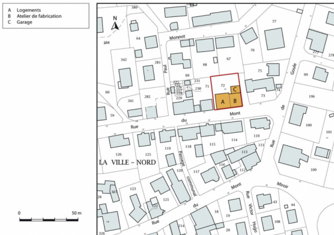
Plan-masse et de situation. Extrait du plan cadastral, 2015, section AB. 25, Maïche, 27 et 29 rue du Mont
