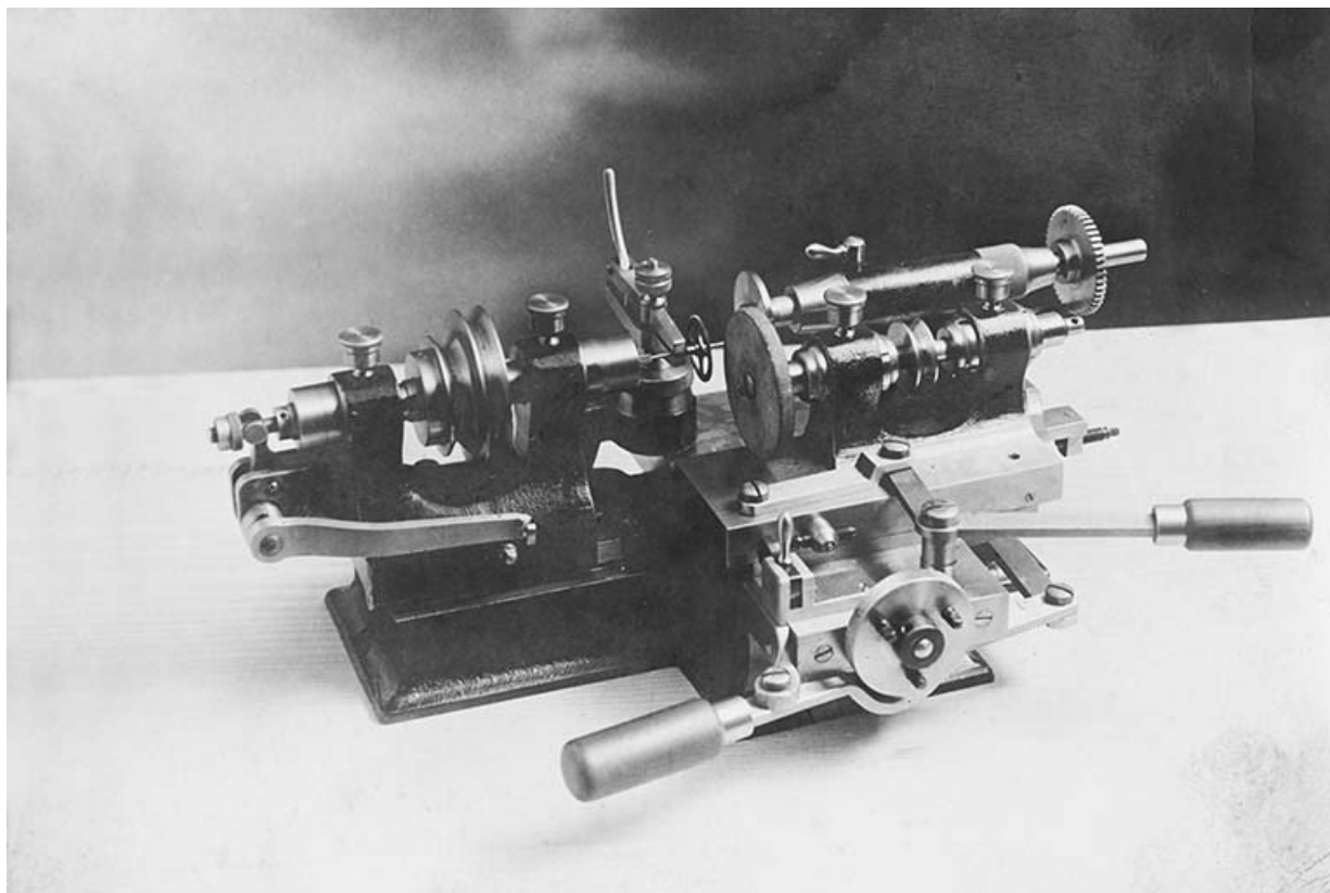
[Machine à rectifier les siettes ?], 2e quart 20e siècle ? (après 1936). 25, Maïche, 13 rue Sous Montjoie
