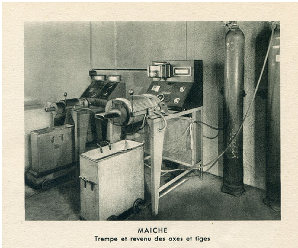
Maïche. Trempe et revenu des axes et tiges, 1950.
