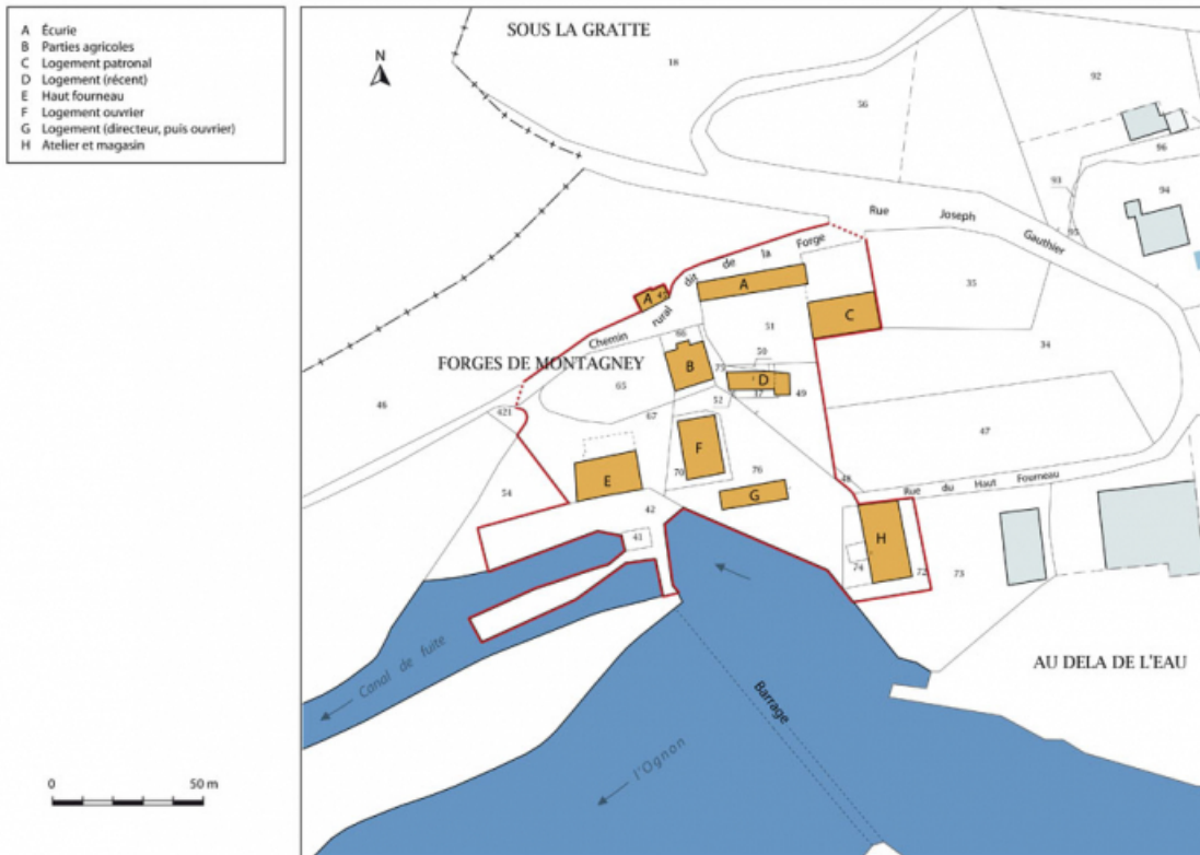
Plan-masse et de situation. Extrait du plan cadastral, 2015, section C. 25, Montagney-Servigney rue du Haut fourneau
