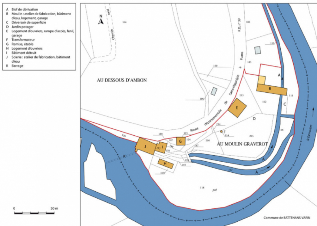
Plan-masse et de situation. Extrait du plan cadastral, 2015, section B. 25, Cour-Saint-Maurice, lieudit : le Moulin du Bas
