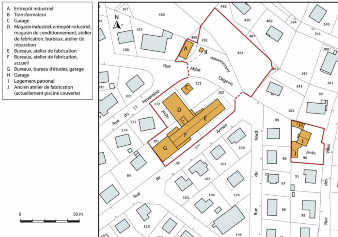
Plan-masse et de situation. Extrait du plan cadastral, 2015, section AB. 25, Charquemont, 9 rue de la 1ère Armée
