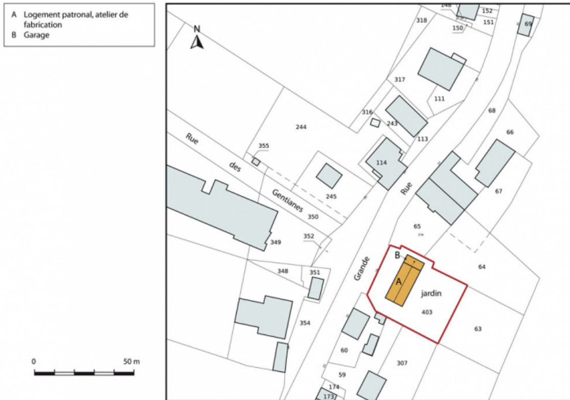
Plan-masse et de situation. Extrait du plan cadastral, 2013, section AC. 25, Les Écorces, 19 Grande Rue
