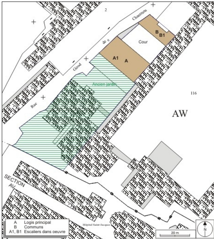
Plan masse et de situation. Extrait du plan cadastral, 1974, section AW. 25, Besançon, 9 rue Girod de Chantrans, lieudit : îlot Saint-Jacques
