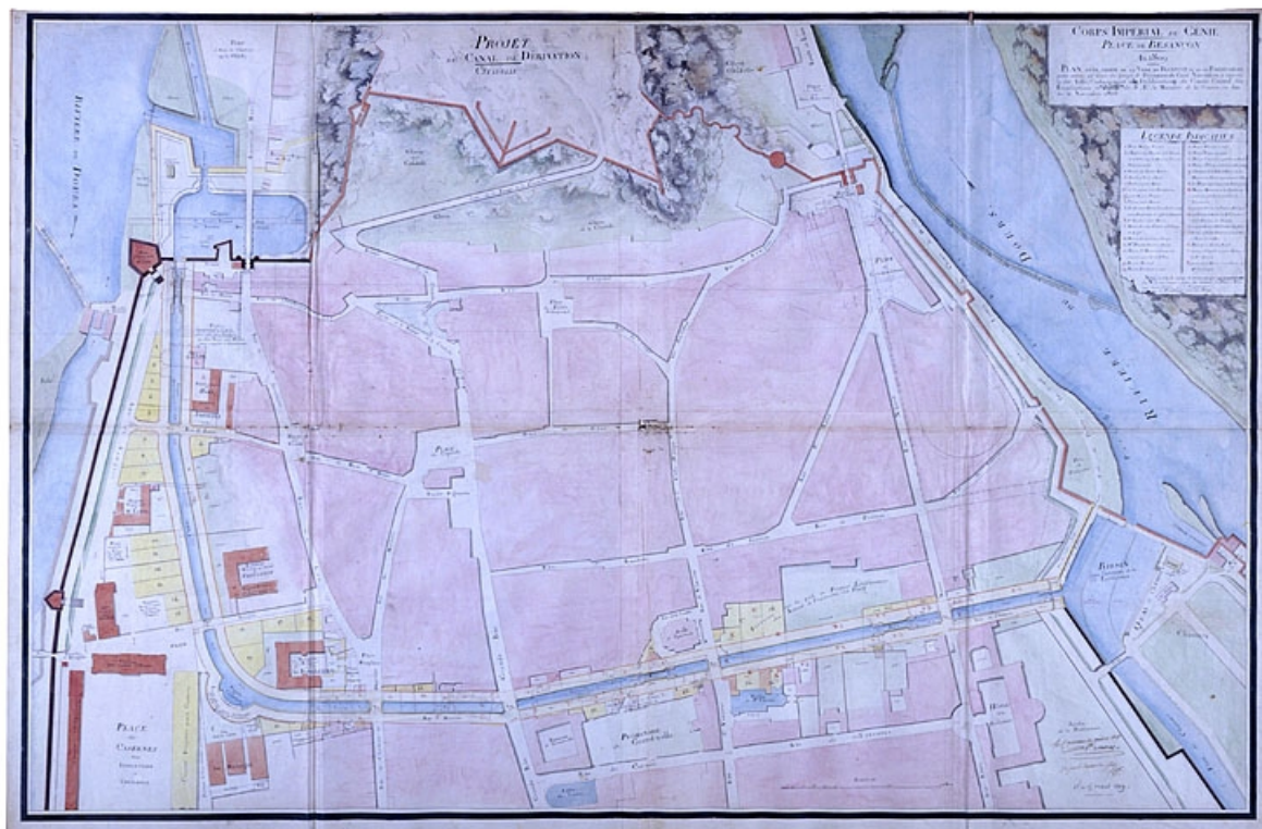
Plan d'une partie de la cité de Besançon et de ses fortifications, pour servir au projet du tracé de dérivation du canal Napoléon à travers ladite ville, 1809.
