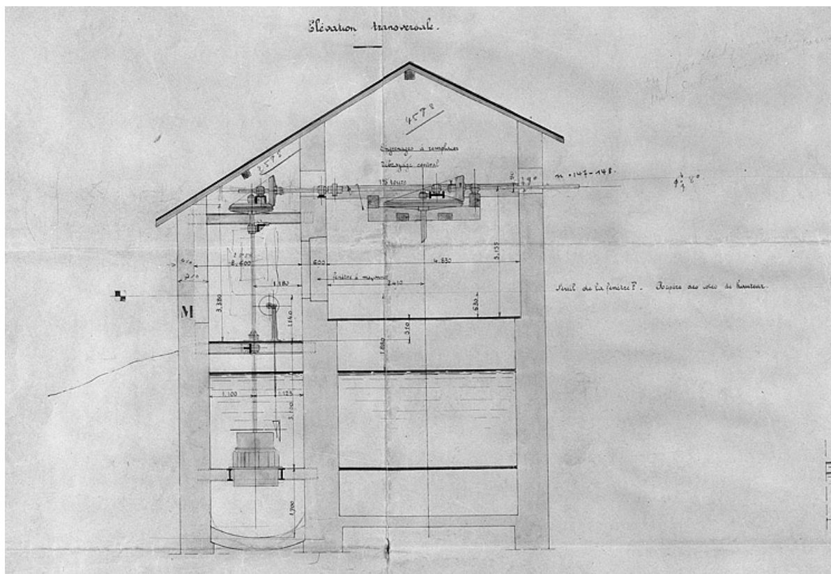
Projet d'installation d'une turbine Hercule-Progrès (Ets Singrün à Epinal), élévation transversale.
