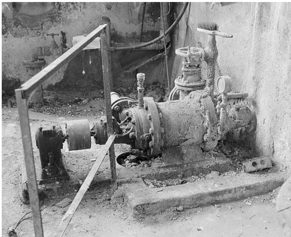
Pompe Sulzer, placée dans l'atelier de mécanique, permettant d'alimenter l'usine en eau depuis un réservoir placé à l'extérieur. 25, Baume-les-Dames rue des Pipes, lieudit : Gondé
