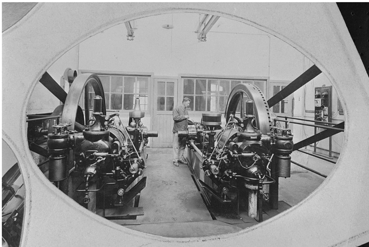
Salle des machines : moteurs à gaz pauvre.
