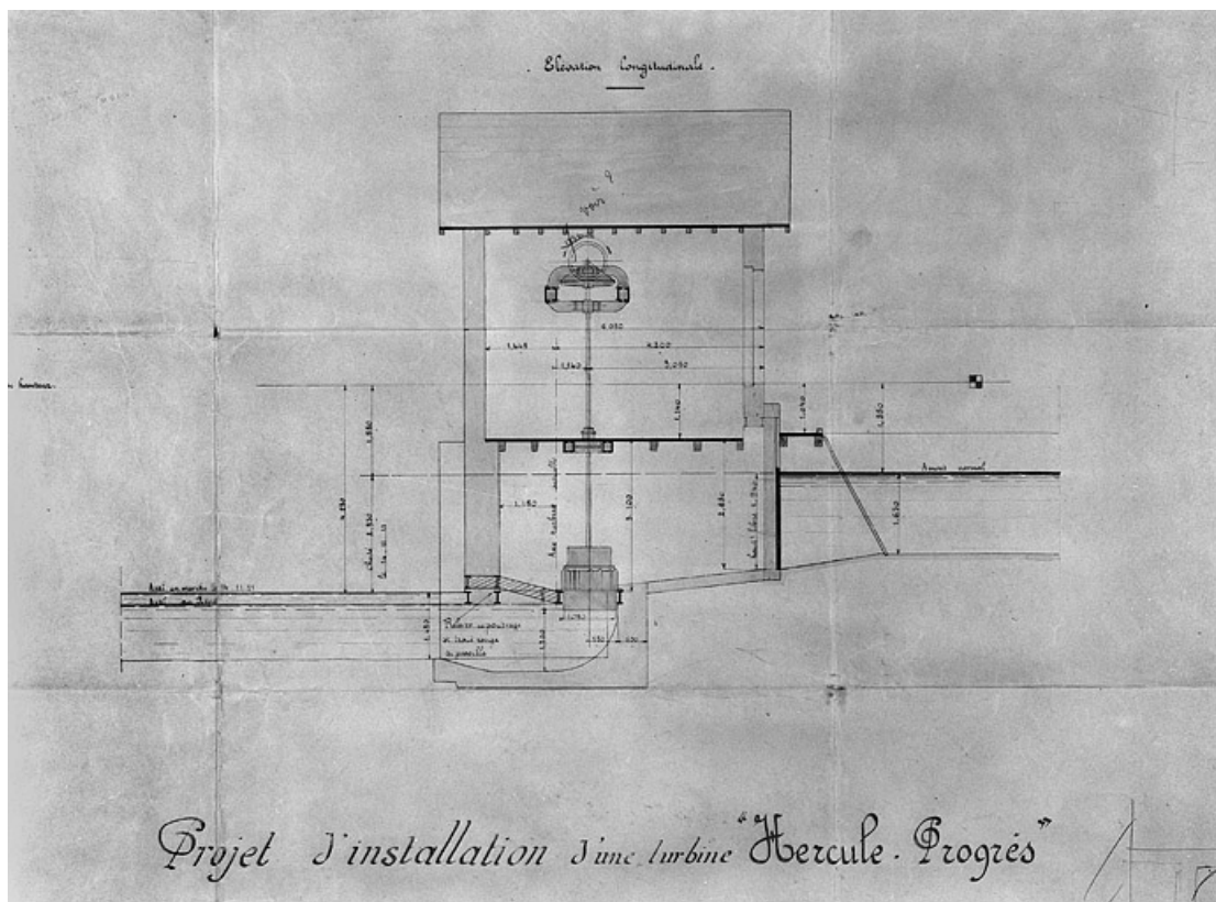
Projet d'installation d'une turbine Hercule-Progress (Ets Singrün à Epinal), élévation longitudinale.
