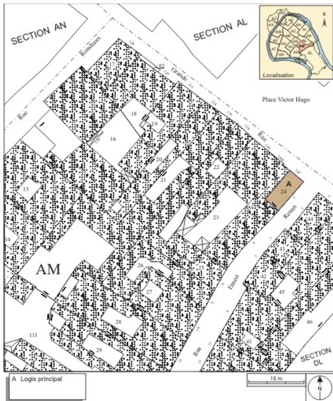
Plan masse et de situation. Extrait du plan cadastral, 1974, section AM. 25, Besançon, 2 rue Renan, lieudit : îlot Ronchaux
