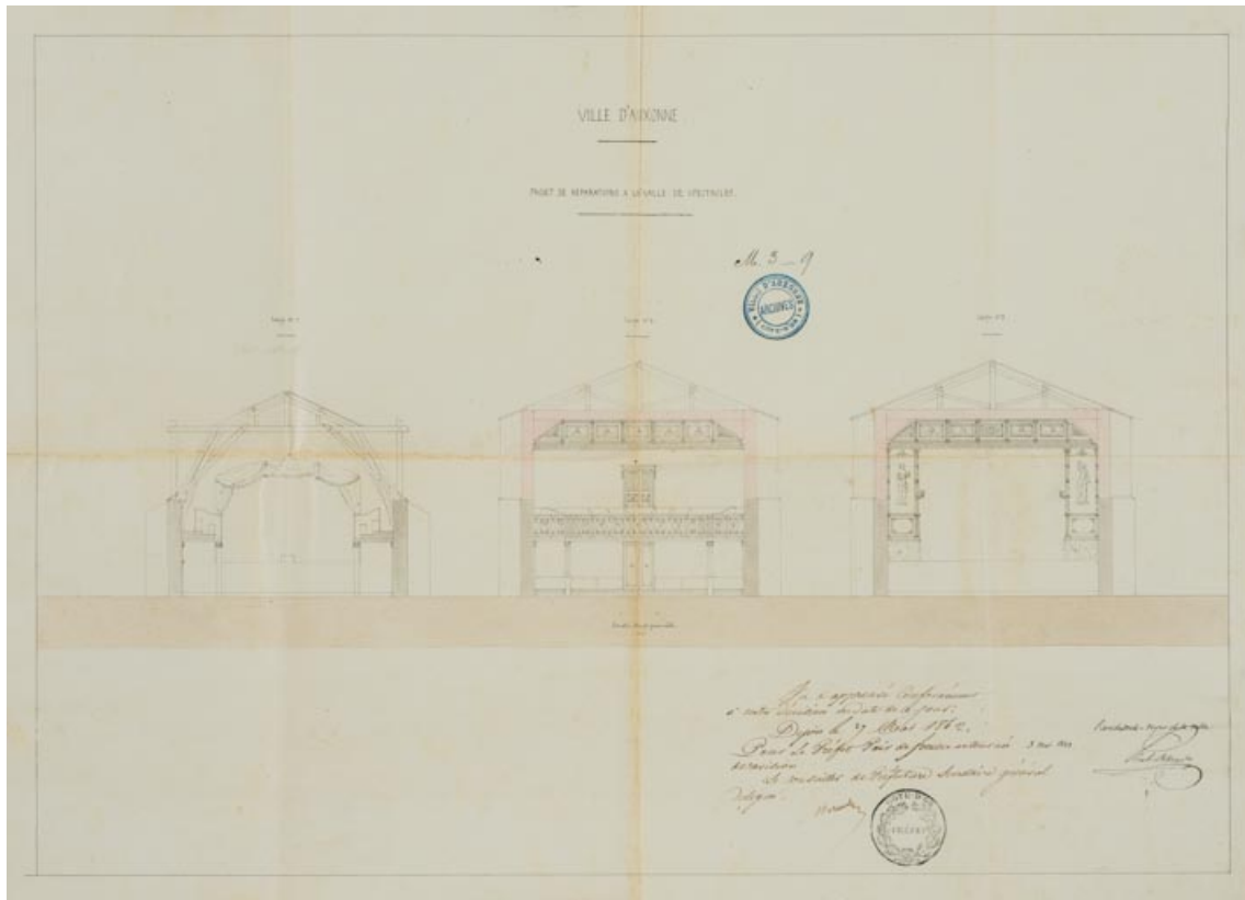
Ville d'Auxonne. Projets de réparations à la salle de spectacle. [Coupe transversale]. 3 mai 1842. 21, Auxonne boulevard Pasteur
