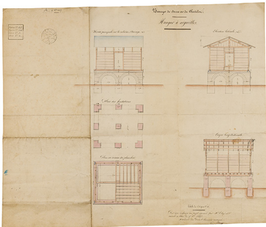
Barrages de Seurre et du Châtelet. Hangar à aiguilles. [Plan, coupe et élévation]. 17 octobre 1847. 21, Pagny-la-Ville, lieudit : PK 200
