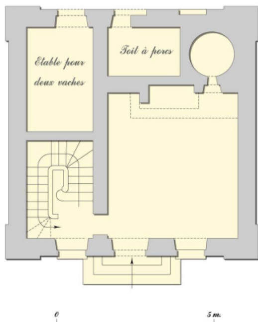
Maison d'éclusier par l'ingénieur Perronet, d'après un document ancien, plan du rez-de-chaussée.
