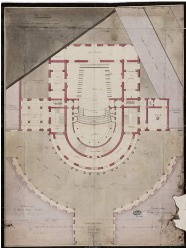
Plan du rez de chaussée de la salle de spestacle [sic] projetée sur l'emplacement du terrain appartenant à la ville [... Variante du 3e projet de Cellierier à l'emplacement du couvent des jacobines]. S.d. [1787].
