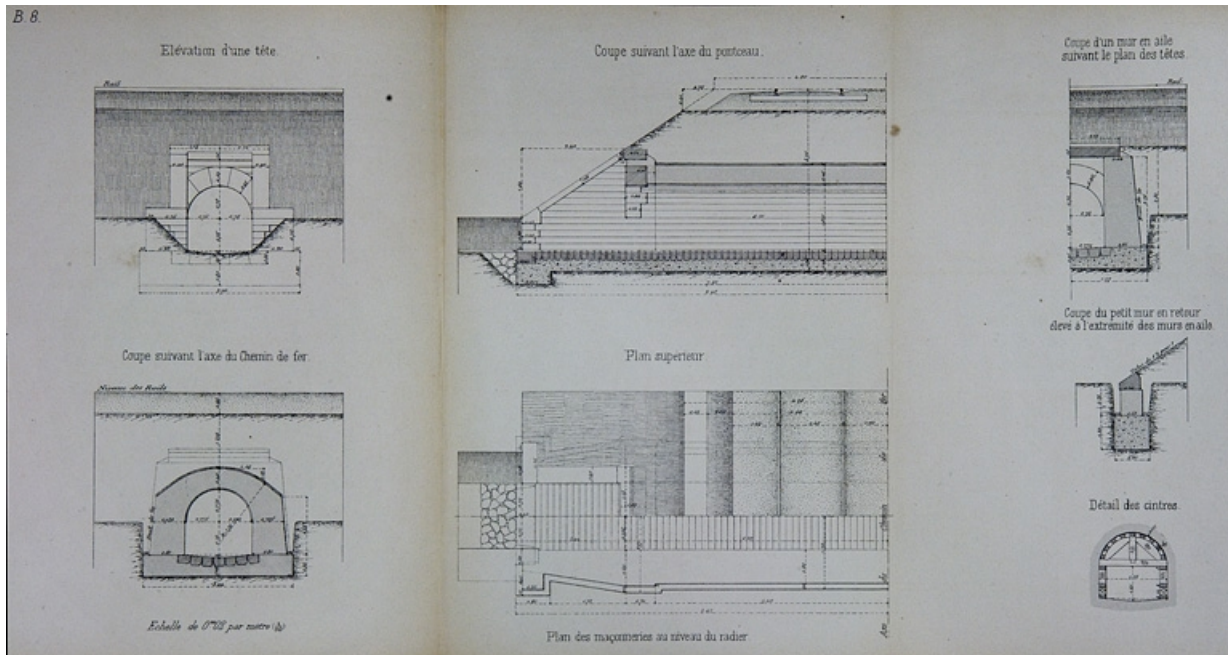
Aqueduc voûté de 1 m 50 d'ouverture. Type de la Cie Paris - Lyon Méditerranée. B 8 [plan, coupes et élévation], 1879.
