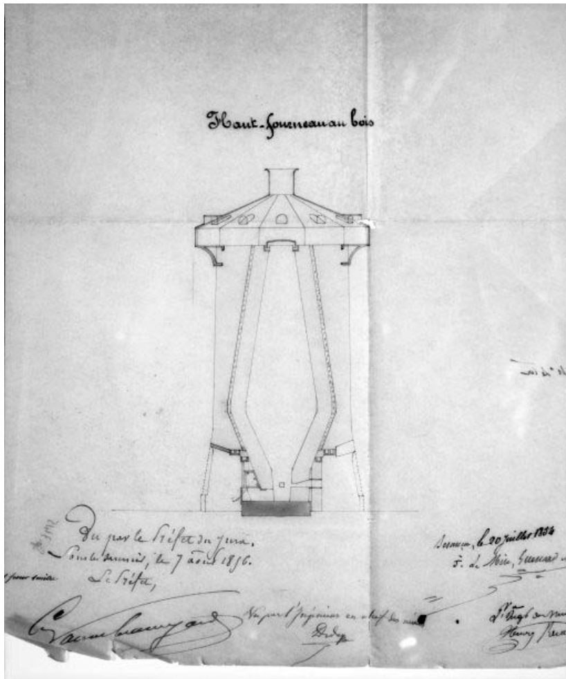
Coupe d'un haut-fourneau au bois. 39, Rans
