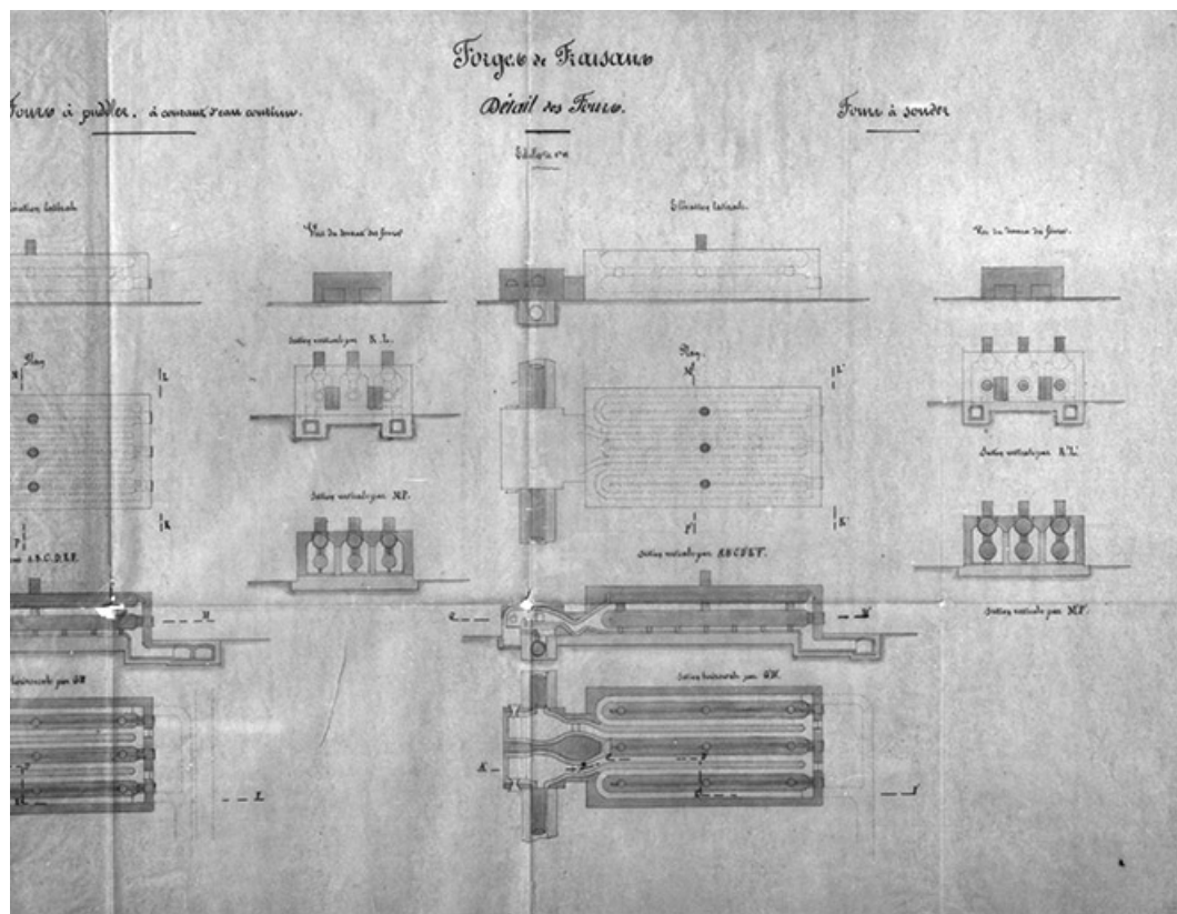
Usine de Fraisans. Détail des fours [les fours à souder].
