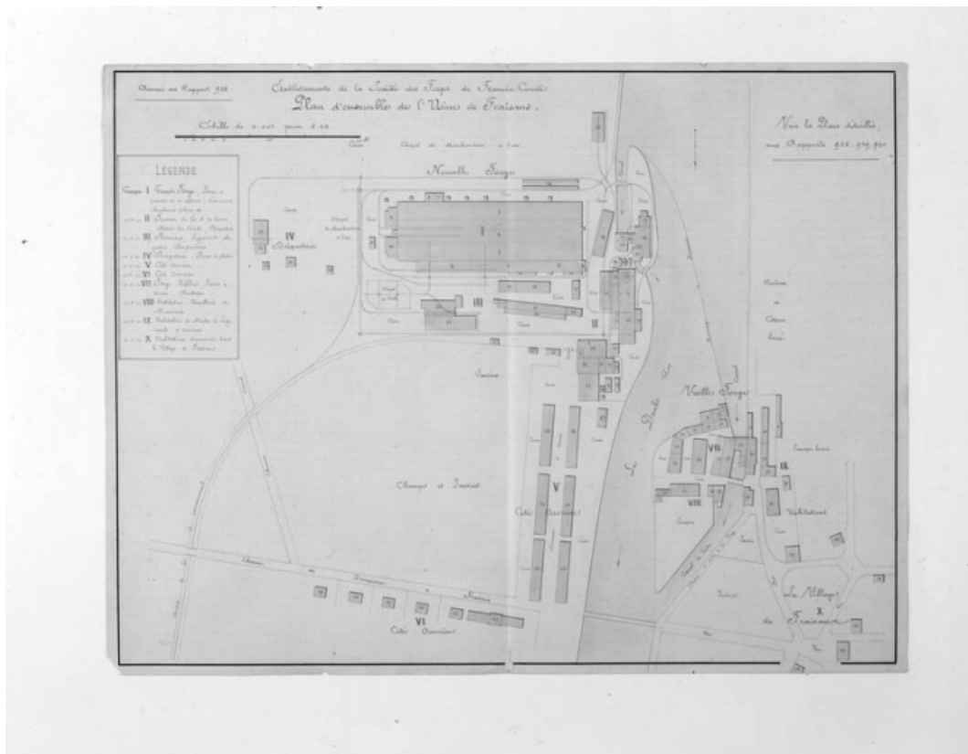
Etablissements de la Société des Forges de Franche-Comté. Plan d'ensemble de l'Usine de Fraisans. 39, Fraisans rue de la Gare
