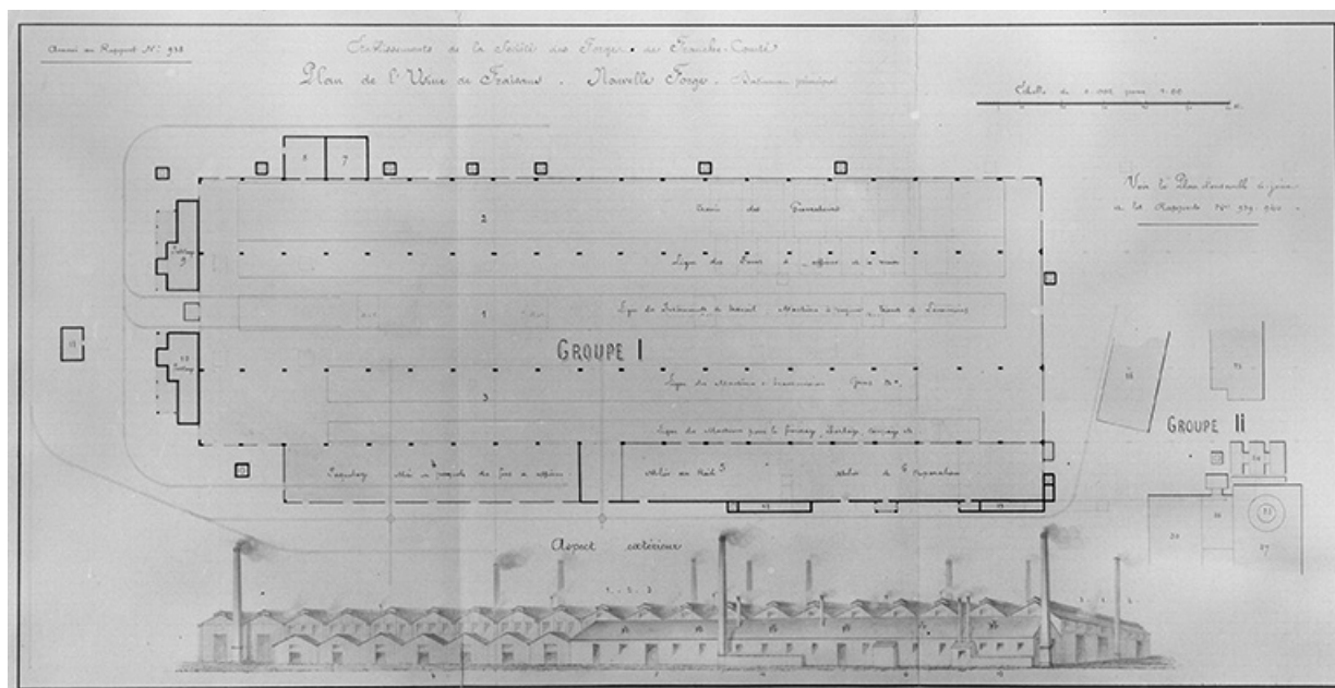
Etablissements de la Société des Forges de Franche-Comté. Plan de l'Usine de Fraisans. Nouvelle Forge. Bâtiment principal. 39, Fraisans rue de la Gare
