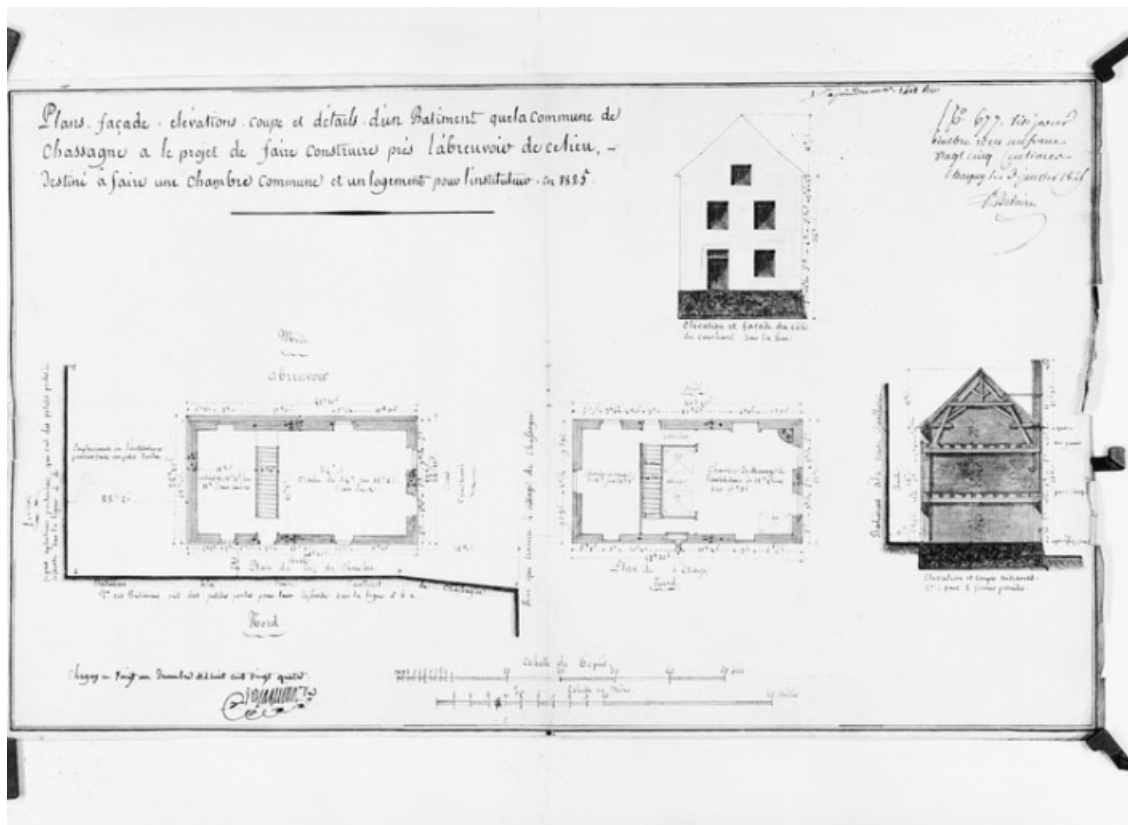
Projet de mairie-école daté 1824 (non réalisé). Dessin aquarellé par Jaquinot J.D. père (architecte). 21, Chassagne-Montrachet
