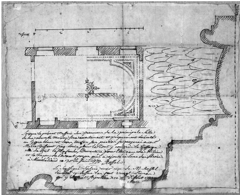
Plan du décor du plafond du grand salon, coupes des moulures, détail de la frise, 1773. 25, Montbéliard, 8 place Saint-Martin
