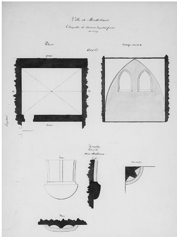
Chapelle. Plan, coupe et relevés des ogives, vers 1866. 25, Montbéliard, 3 rue du Château
