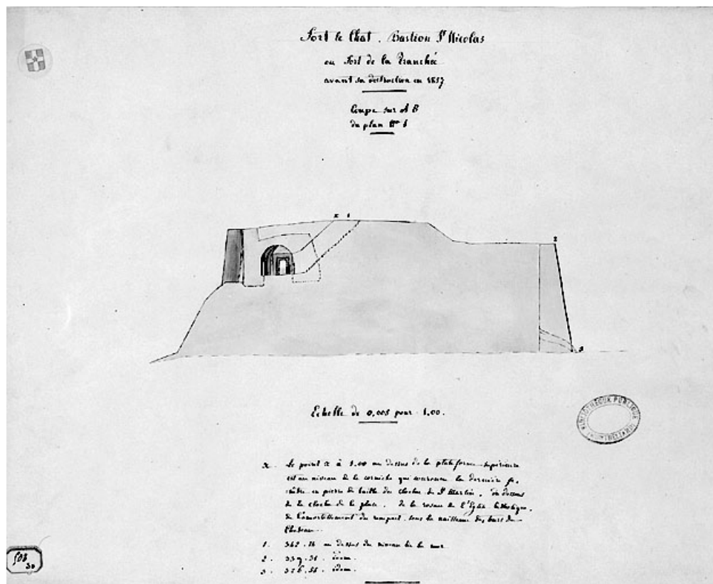
Fort Le Chat. Bastion St-Nicolas. Coupe transversale, 1ère moitié 19e siècle. 25, Montbéliard rue Aristide Briand
