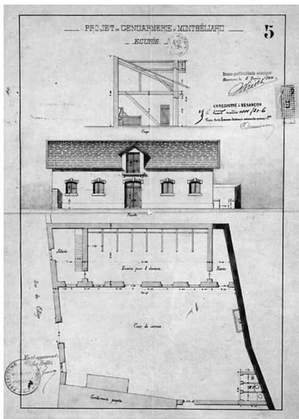
Projet de Gendarmerie à Montbéliard. Ecuries, 1888. 25, Montbéliard, 6 rue de Velotte
