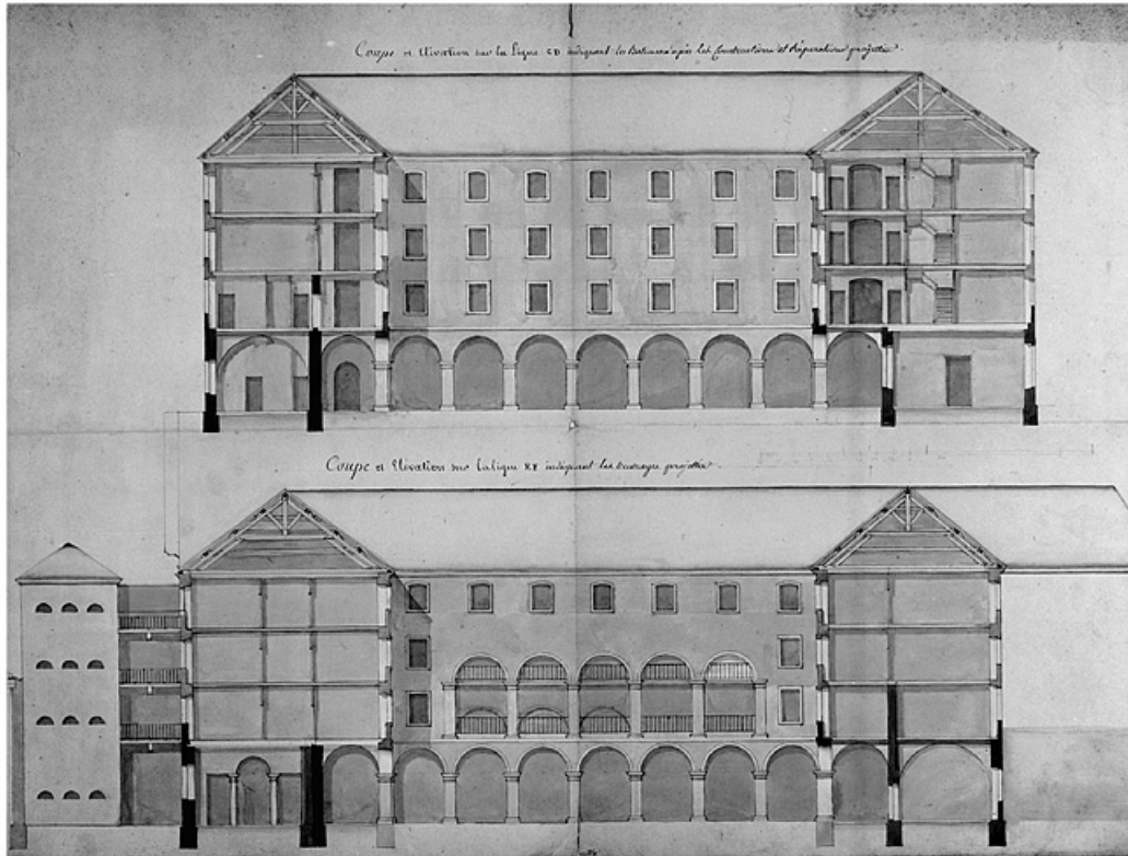
Elévations des façades des bâtiments conventuels après transformation en séminaire (projet de transformation). 39, Lons-le-Saunier rue des Cordeliers
