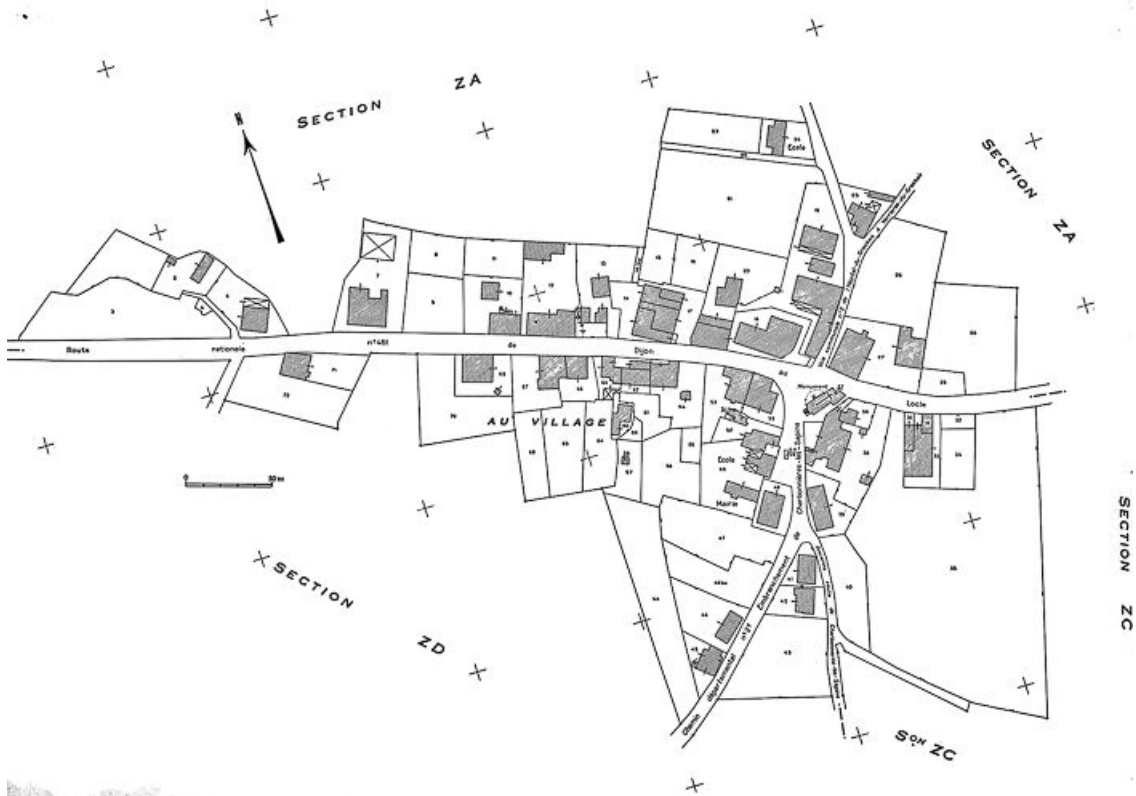
Plan cadastral, 1968, section AB, échelle 1 : 1000. 25, L'Hôpital-du-Grosbois
