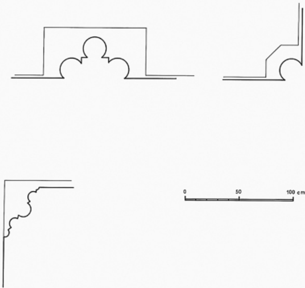
Détail : coupe des colonnes par J.-M. Demoly et Gilbert Poinsot, 1975.
