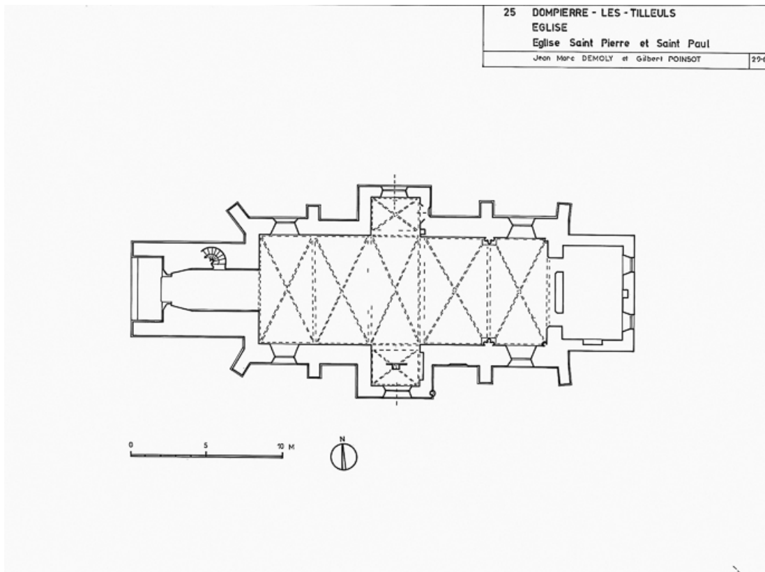
Plan au sol par J.-M. Demoly et Gilbert Poinsot, 1975.
