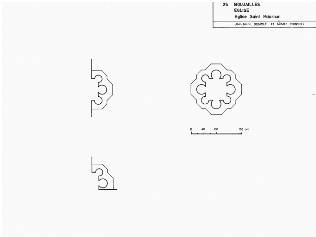
Plan des petits piliers : relevé-croquis J.-M Demoly et Gilbert Poinso, 1975. 25, Boujailles place de l' Eglise
