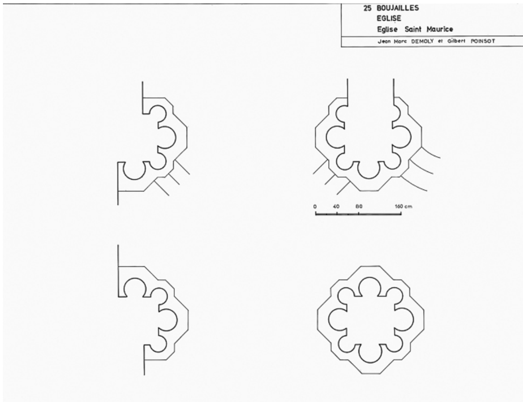
Plan des gros piliers : relevé-croquis J.-M Demoly et Gilbert Poinso, 1975.t, 1975. 25, Boujailles place de l' Eglise
