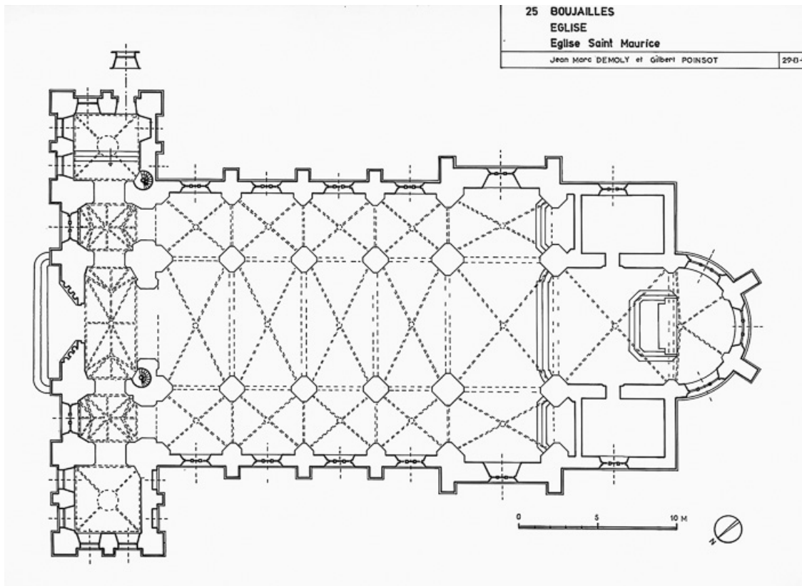
Plan au sol : relevé-croquis J.-M. Demoly et Gilbert Poinsot, 1975.
