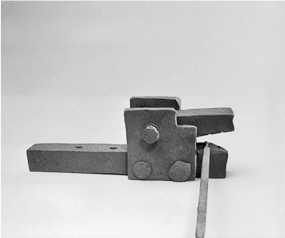
Cloutière avec un bâton de section carré servant à la fabrication des pointes de toupie ("fiardes").
