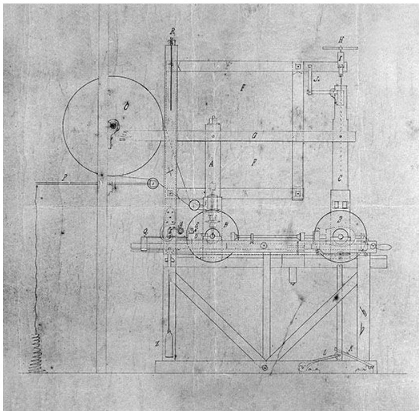
Elévation de la face latérale gauche.
