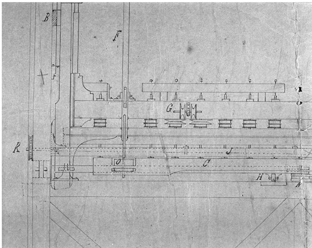
Élévation de la face postérieure : détail de la partie gauche du plan.
