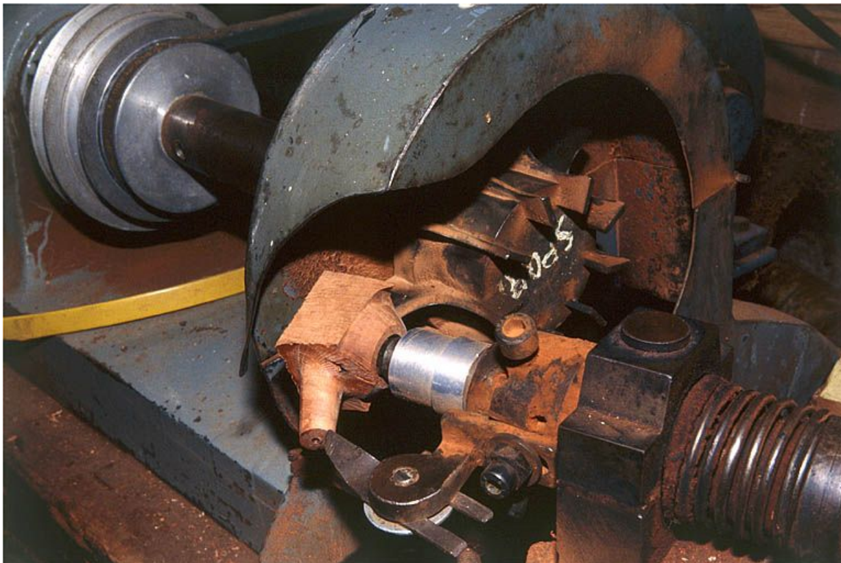
Mandrin conique et fraise.
