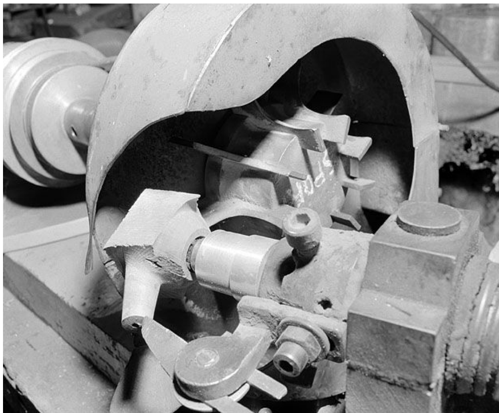
Mandrin conique et fraise.
