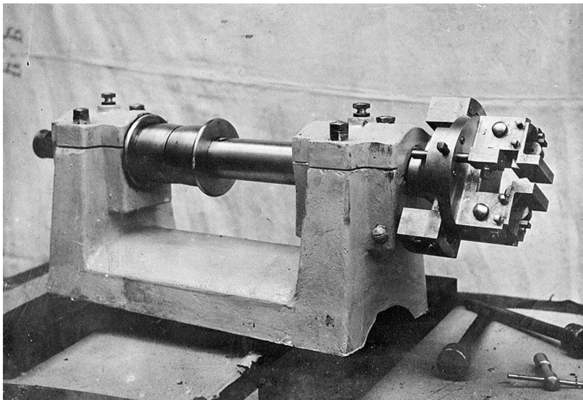
Exemple de tour de pipier, avec mandrin gueule de loup, du constructeur mécanicien Lizon.
