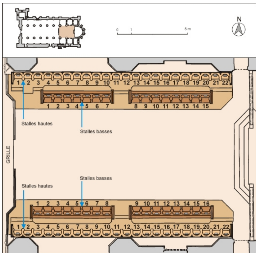
Plan de situation et plan général des stalles.
