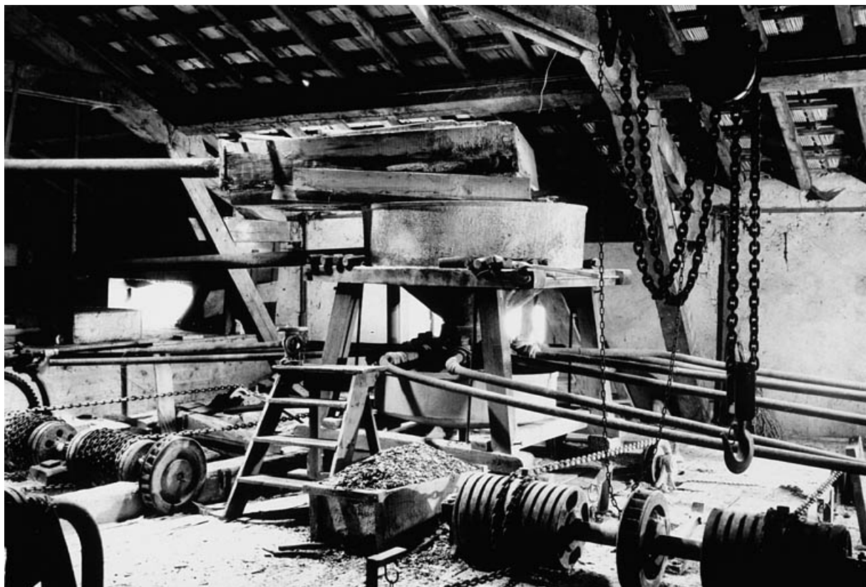
Système de distribution du mélange eau-sable : vue d'ensemble. Distributeur centrifuge surmonté d'un tamis en bois. 39, Saint-Amour, 2 à 6 rue de la Marbrerie
