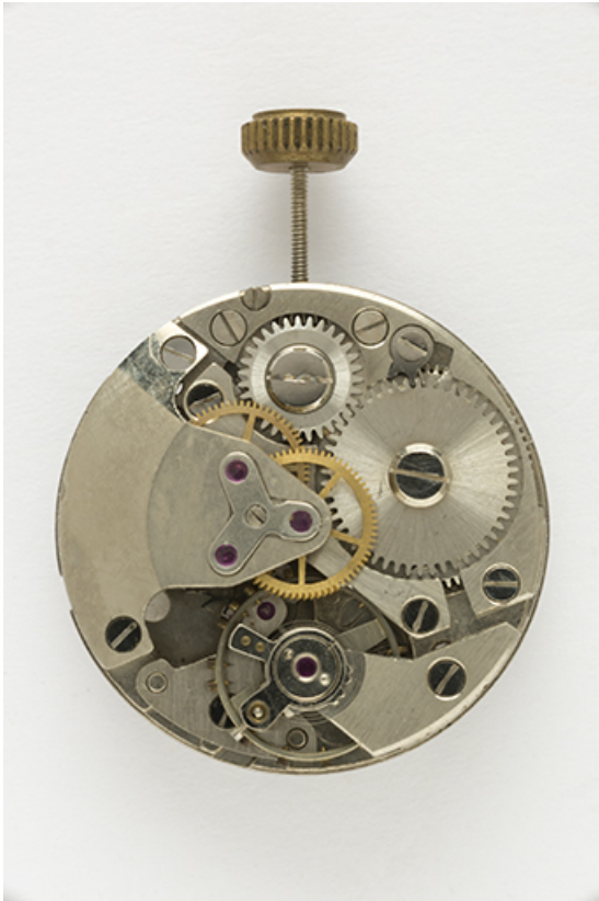
Mouvement Parrenin HP 90 : face côté ponts.
