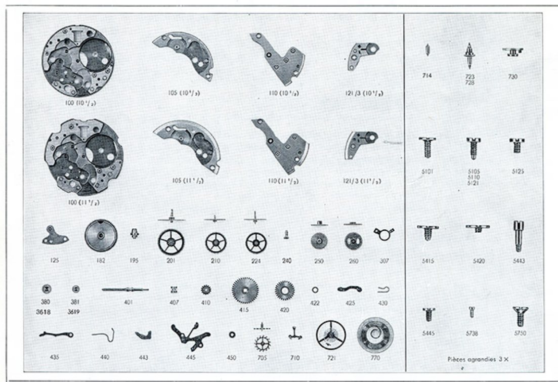
Calibre 10 1/2 - 11 1/2''' - 233-68 - fournitures du calibre de base, 1973. 25, Maîche
