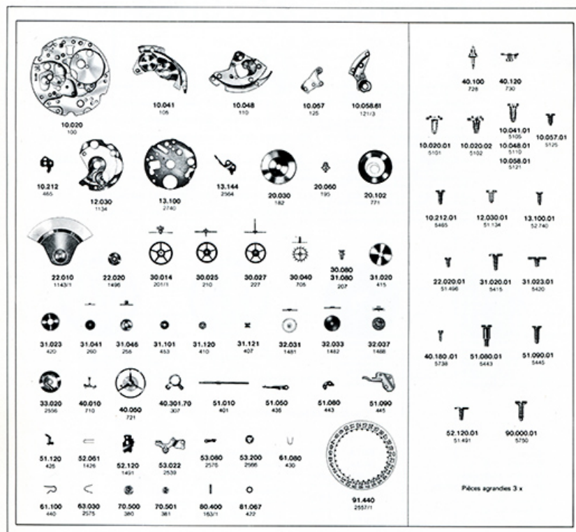
Calibre 11 1/2''' - 4611 A Automatique Calendrier [éclaté des fournitures], 1973. 25, Maîche
